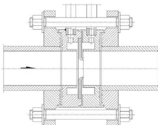
1/4 圆喷嘴 1/4 rond Nozzle
